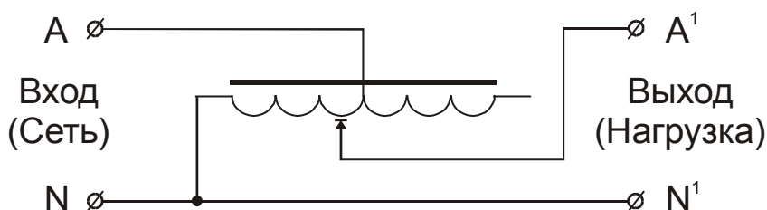
Рис.1 Схема включения автотрансформатора
